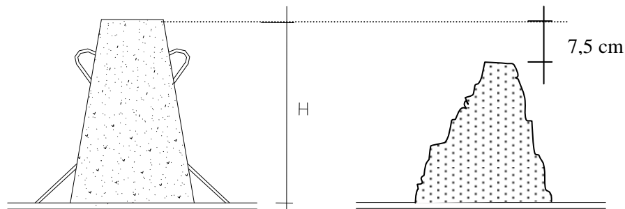
Gambar 6 Tinggi Slump Test Hasil Pengujian
