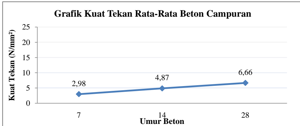
Gambar. 6 Grafik Hubungan Kuat Tekan Rata-Rata Beton Dengan Campuran Cangkang Buah Sawit Berbentuk Silinder Terhadap Umur Beton
