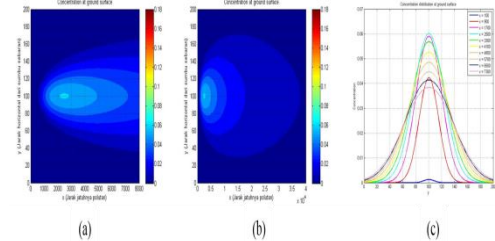
Gambar 5. Untuk H = 70 , (a) dengan x = 8000\text{m} , (b) dengan x = 40000 m serta (c) grafik distribusi konsentrasi polutan
