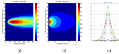
Gambar 2. Untuk H = 40 , (a) dengan x = 3000\text{m} , (b) dengan x = 20000\text{m} serta (c) grafik distribusi konsentrasi polutan.
