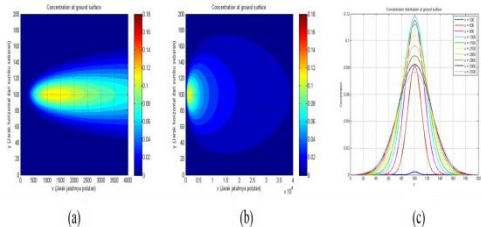
Gambar 3. Untuk H = 50 , (a) dengan x = 4000\text{m} , (b) dengan x = 40000\text{m} serta (c) grafik distribusi konsentrasi polutan
