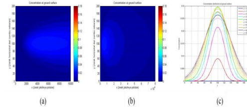
Gambar 7. Untuk H = 100 , (a) dengan x = 10000\text{m} , (b) dengan x = 80000 m serta (c) grafik distribusi konsentrasi polutan
