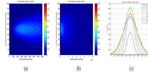
Gambar 6. Untuk H = 80 , (a) dengan x = 8000\text{m} , (b) dengan x = 80000 m serta (c) grafik distribusi konsentrasipolutan
