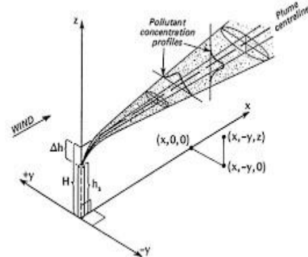
Gambar 1. Pola sebaran asap dengan dispersi Gauss
